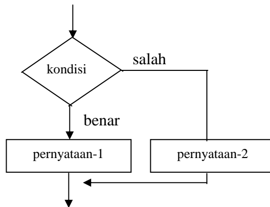
Gambar 5.2. Diagram alir if-else
